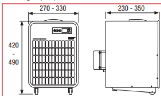
Afmetingen (mm)
